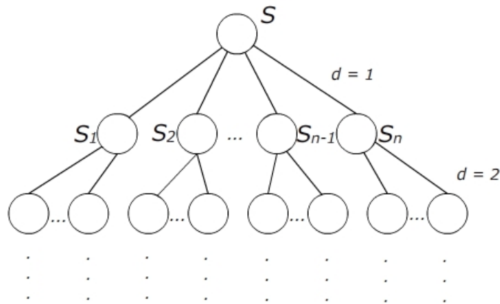
Figuur 5: Monte Carlo spelboom
